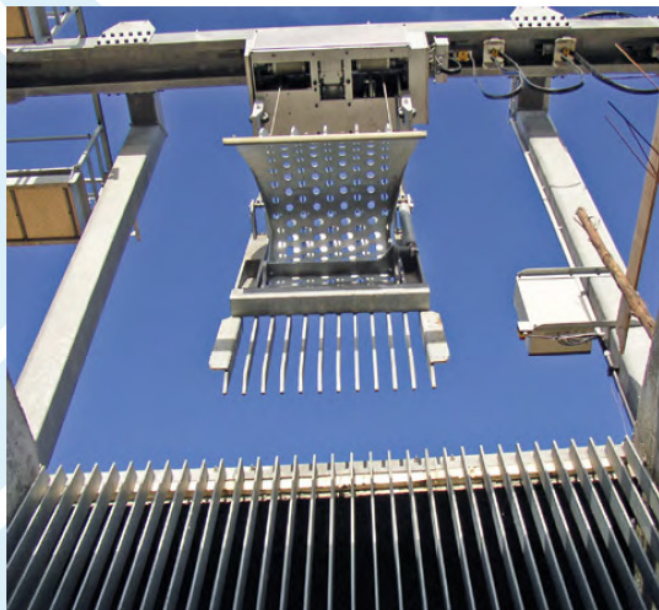
Dégrilleur à poche
